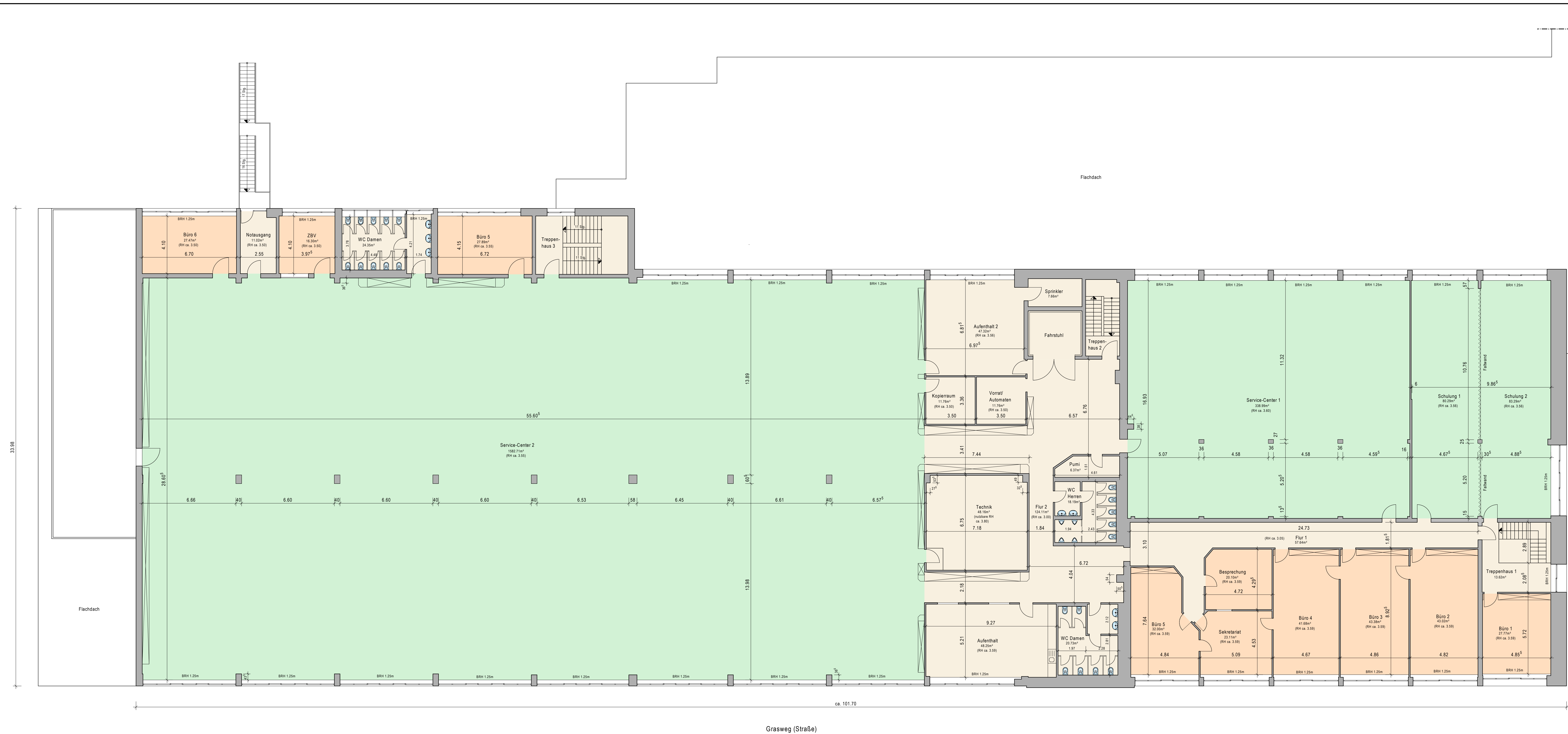
OBERGESCHOSSGRUNDRISS
